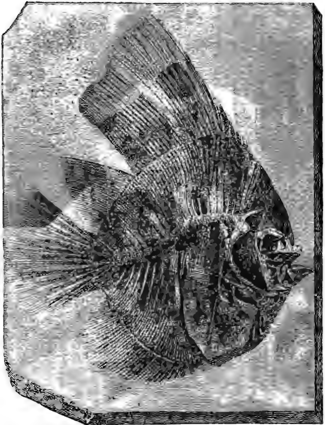
PLATAX ALTISSIMUS. A Ctenoid of Monte Bolca. ( Eocene. )
